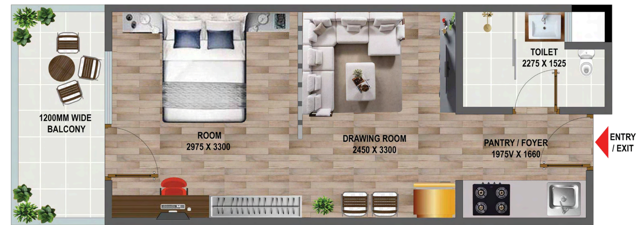
Suite Plan B
