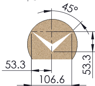
DETALLE A ESCALA 1 : 6
