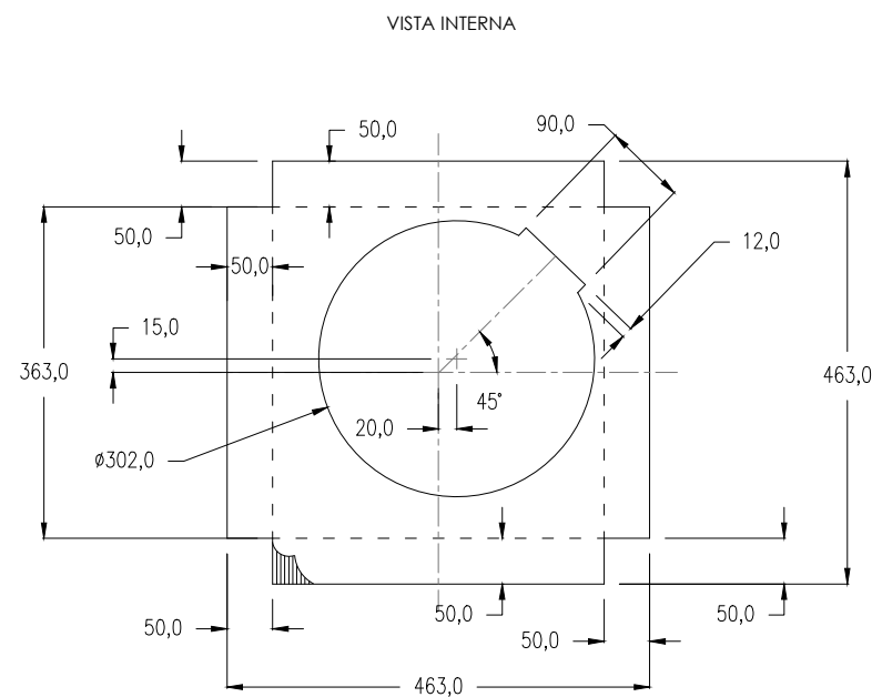
ACCESORIO INTERIOR DOS PIEZA POR JUEGO
