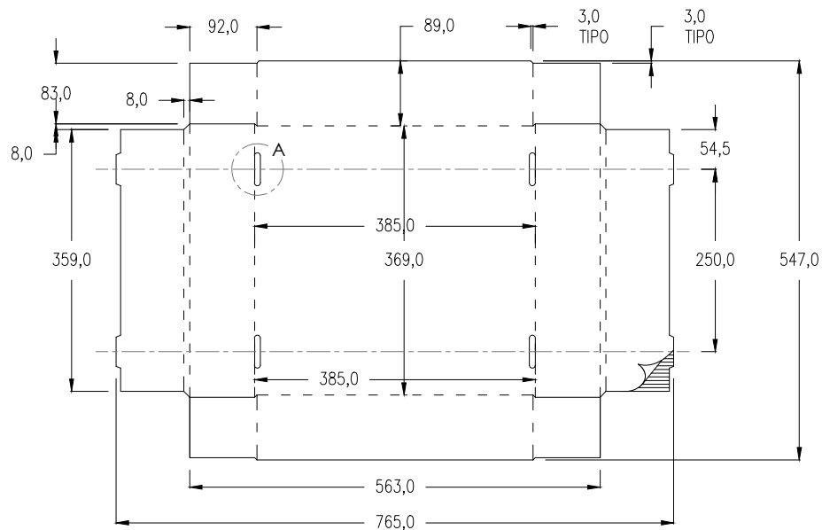
DISEÑO ESTRUCTURAL VISTA INTERNA DE TAPA Y BASE
