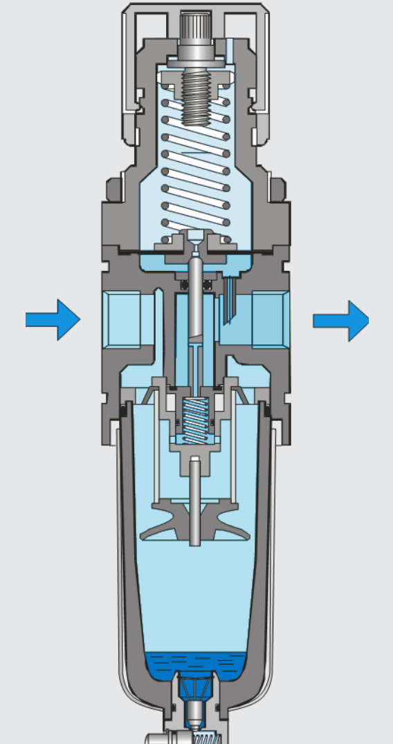
Filtro-regulador
