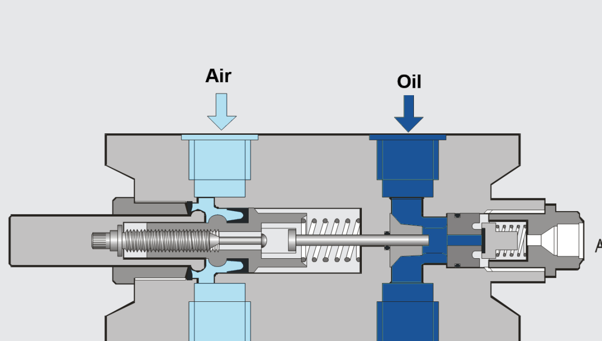
Lubricador por inyección
