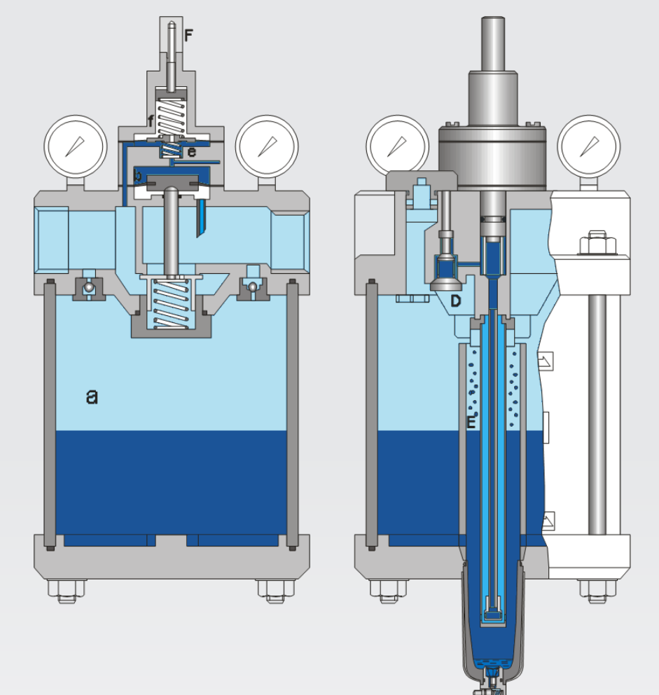
Unidad de lubricación centralizada
