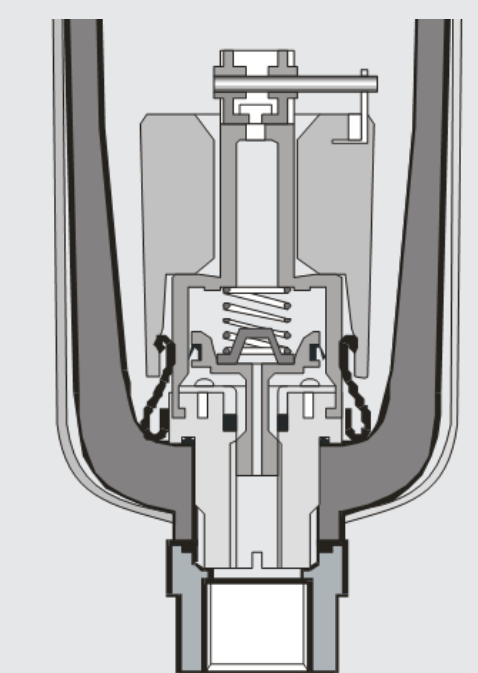
Purga automática
