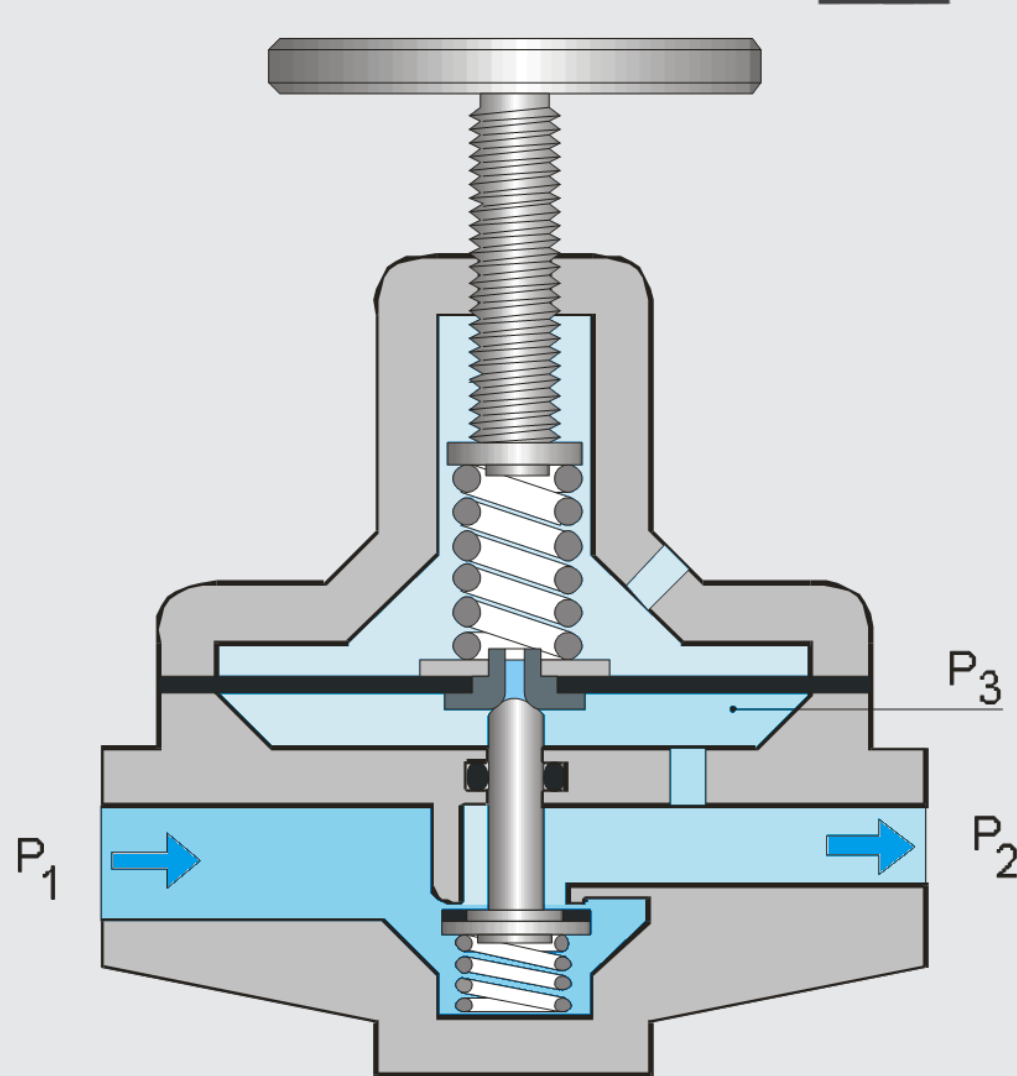
Regulador de presión estándar
