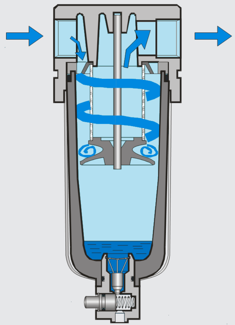
Filtro estándar
