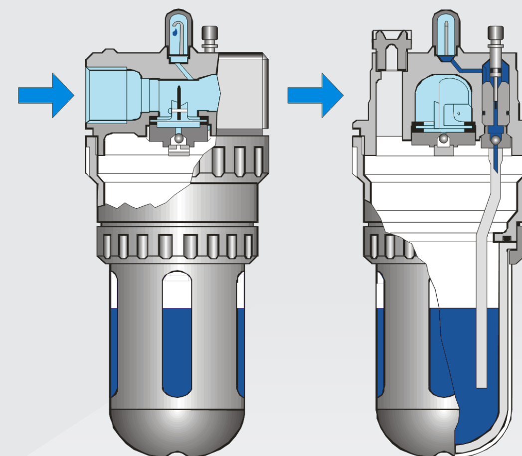
Lubricador de microneblina
