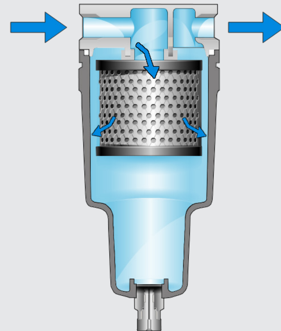
Filtro submicrónico
