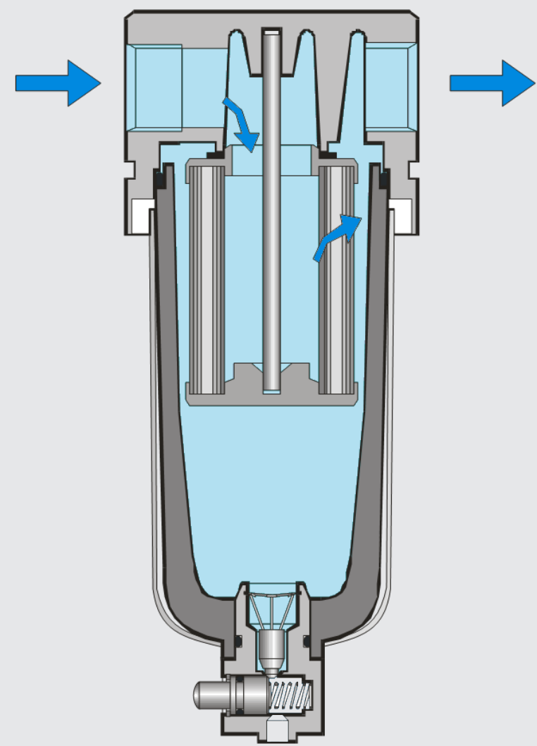
Filtro micrónico
