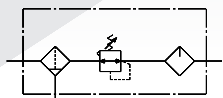
Unidad de tratamiento de aire
