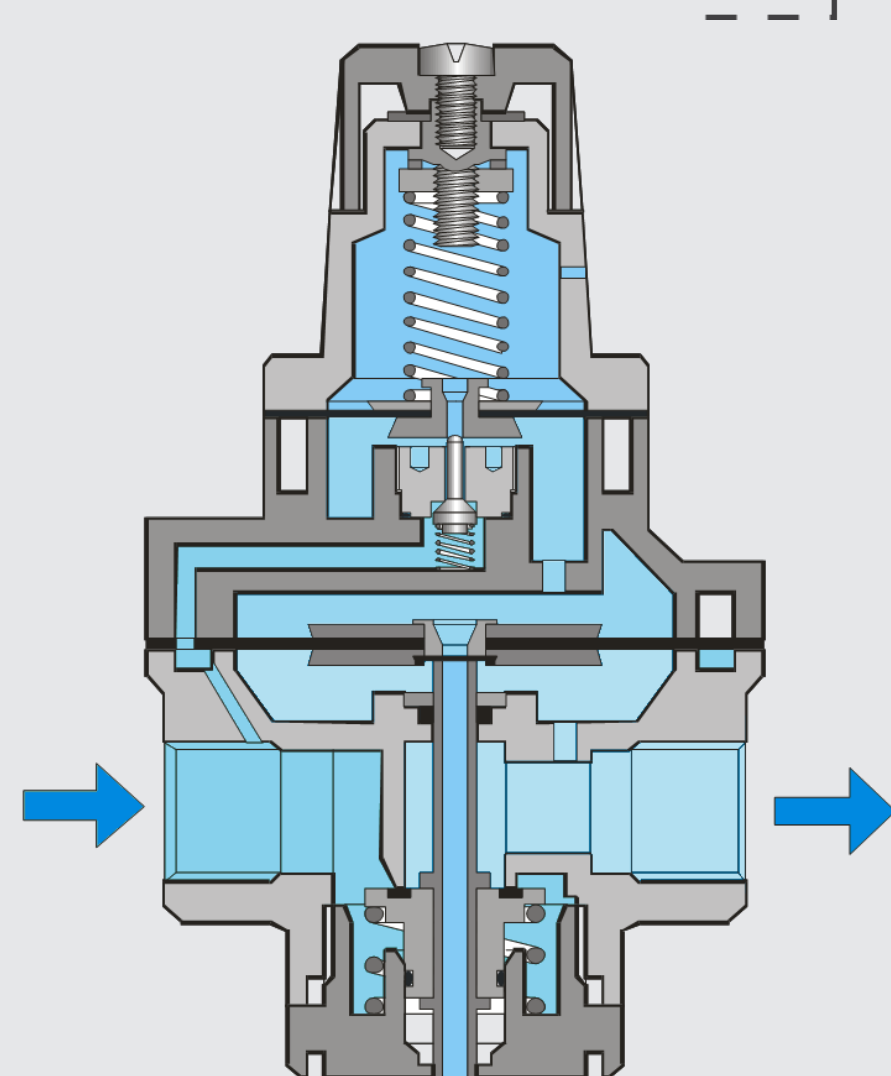
Regulador de presión pilotado
