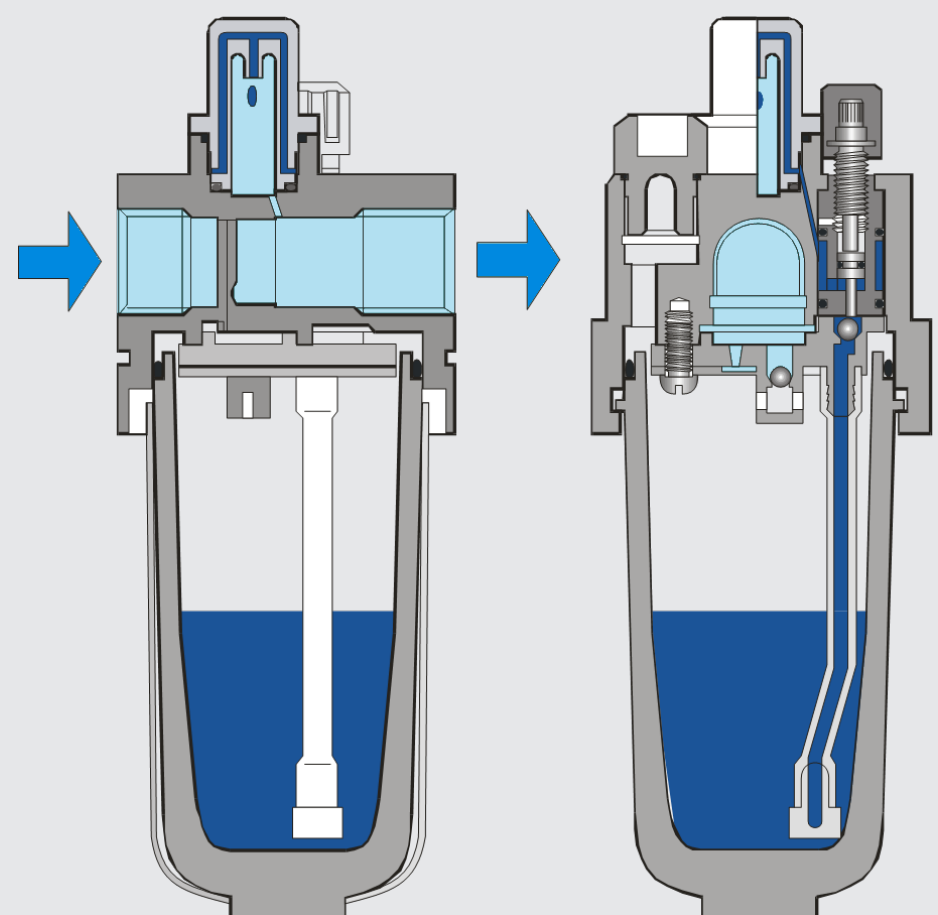
Lubricador proporcional
