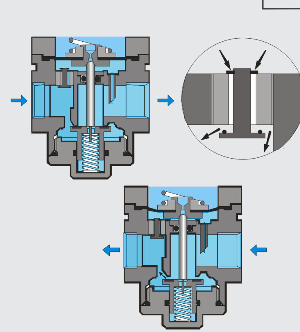
Regulador de presión con antirretorno
