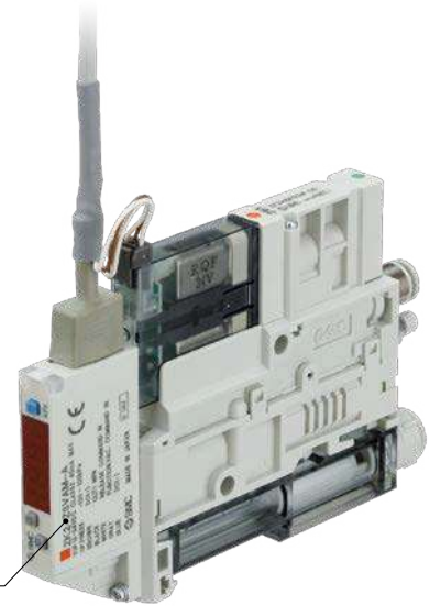
Presostato digital para vacío con función de eficiencia energética
