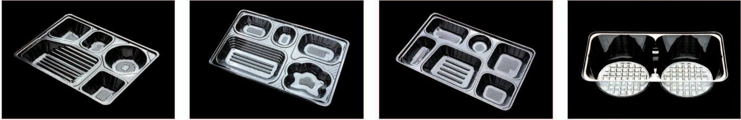
名 称:LGD 材质:OPS 名 称:LGN 材质:OPS 名 称:LGR 材质:OPS 名 称:36G饼干盒 材质:OPS 模具编号:RZ-27 模具编号:RZ-29 模具编号:RZ-28 模具编号:RZ-23 制品尺寸:279×172 克重:4.6g 制品尺寸:255×155×30 克重:5.4g 制品尺寸:269×164×30 克重:5.4g 制品尺寸:107×57×28.5 克重:1.2g 纸箱尺寸:510×420×240 入箱数:3000枚 纸箱尺寸:485×450×275 入箱数:3000枚 纸箱尺寸:515×460×290 入箱数:3000枚 纸箱尺寸:520×480×435 入箱数:14400枚
