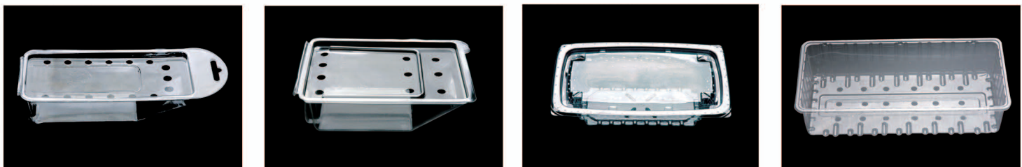
名称:辣椒盒 模具编号:RZ-90 制品尺寸:473×86×57 纸箱尺寸:600×472×445 材质:PET 克重:30g 入箱数:400枚 名称:T型西红柿盒 模具编号:RZ-73 制品尺寸:342×133×51.5 纸箱尺寸:760×365×600 材质:PET 制品克重:26.5g 入箱数:600枚 名称:NO-100 模具编号:RZ-85 制品尺寸:身175×105×46 盖171×101×10 纸箱尺寸:盖700×530×520 身630×370×540 克重:身8.8g 盖5.8g 入箱数:盖2000枚 身1000枚 材质:PET 克重:17g 入箱数:1000枚 名称:1.5LB黄瓜托盒 模具编号:RZ-108 制品尺寸:254×124×58 纸箱尺寸:575×445×535 材质:PET 克重:17g 入箱数:1000枚
