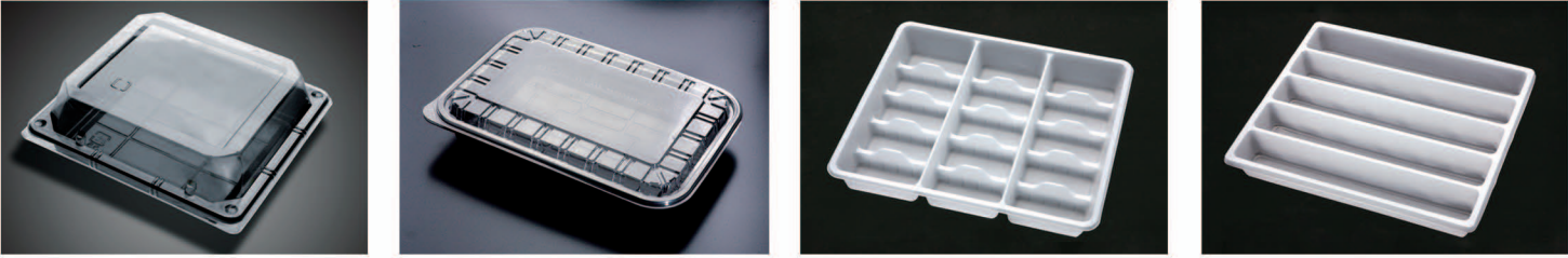
名 称:PP鸡肉盒 模具编号: RZ-59 制品尺寸: 盖208×188×47 身203×185×34 纸箱尺寸: 盖610×445×445 身530×445×445 克 重: 盖13g 身19g 入箱数: 盖800枚 身600枚 材质:盖OPS 身PP 克重: 12. 5g 入箱数: 1250枚 名 称:毛豆盒 模具编号: RZ-24 制品尺寸: 盖285×200×16 身285×200×45 纸箱尺寸: 盖600×580×405 身600×580×405 克 重: 盖27. 5g 身50g 入箱数: 盖800枚 身400枚 材质:盖PET 身PP 克重: 15g 入箱数: 1200枚 名 称:PP15分格 模具编号: RZ-21 制品尺寸: 200×177×30 纸箱尺寸: 535×400×405 材质:PP 克重: 14. 8g 入箱数: 1200枚 名 称:五分格20×25 模具编号: RZ-3 制品尺寸: 210×128×25 纸箱尺寸: 575×445×534 材质:PP 克重: 12g 入箱数: 1250枚
