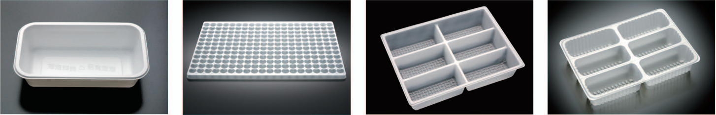
名 称:SG盒 模具编号: RZ-77 制品尺寸: 214. 6×124. 6×52 纸箱尺寸: 760×365×600 材质:PP 克重: 21. 2g 入箱数: 840枚 名 称:PP240格半圆托盘 模具编号: RZ-121 制品尺寸: 550×350×13. 3 纸箱尺寸: 530×405×405 材质:PP 克重: 128g 入箱数: 200枚 名 称:六分格 模具编号: RZ-7 制品尺寸: 180×133×36 纸箱尺寸: 610×445×445 材质:PP 克重: 12g 入箱数: 1200枚 名 称:010-9-1 模具编号: RZ-42 制品尺寸: 185×128×33 纸箱尺寸: 575×445×535 材质:PP 克重: 10g 入箱数: 1200枚
