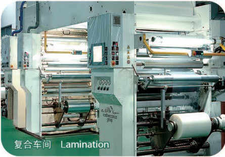
意大利NORDMECCANICA无溶剂复合机, 日本富士产干式复合生产线
