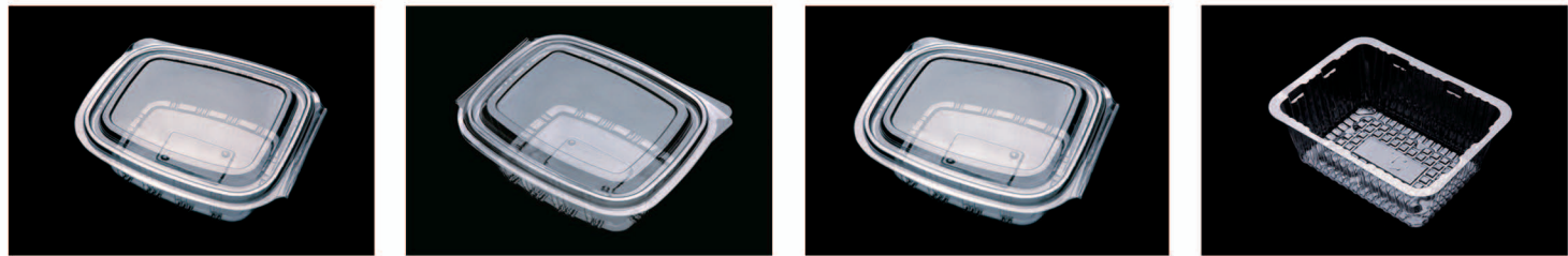
名称:500ml 模具编号:RZ-41 制品尺寸:305×125×53 纸箱尺寸:630×470×400 材质:PET 克重:16.3g 入箱数:600枚 名称:1000ml 模具编号:RZ-33 制品尺寸:385×158×64 纸箱尺寸:520×400×490 材质:PET 克重:28g 入箱数:300枚 名称:750ml 模具编号:RZ-40 制品尺寸:340×138×61 纸箱尺寸:560×350×570 材质:PET 克重:20g 入箱数:400枚 名称:海苔深盒 模具编号:RZ-13 制品尺寸:106×82×45 纸箱尺寸:550×350×510 材质:PET 克重:4.1g 入箱数:2000枚
