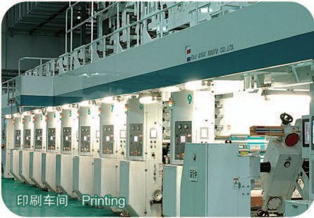
日本富士公司7色, 8色, 9色, 10色高速电子轴凹版印刷机
