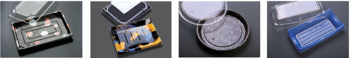
名 称:R2.0寿司盒 材质:盖PET 身HIPS 模具编号: RZ-101 制品尺寸: 身228×154×22盖231×157×32 纸箱尺寸: 身575×445×535 盖575×445×535 克重: 身18.43g 盖14.6g 入箱数: 身600枚 盖400枚 名 称:船型寿司24-15 材质:盖PET 身HIPS 模具编号: RZ02340/S 克重: 身19.4g 盖14g 制品尺寸: 身234×144×27盖237×147×50 名 称:圆盘4.0 材质:盖PET 身HIPS 盖模具号: RZ02350 身模具号: RZ0235S 盖制品尺寸: D322-32 克重: 34.2g 身制品尺寸: D320-30 克重: 50.6g 身盖合装纸箱尺寸: 720X335X335 入箱数: 300枚 名 称: SK-20A 材质: 盖PET 身HIPS蓝 制品尺寸: 191×117×38 克重: 11.7g 模具号: RZ240 纸箱尺寸: 425×380×405 身盖合装纸箱尺寸: 390×435×420 入箱数: 300枚
