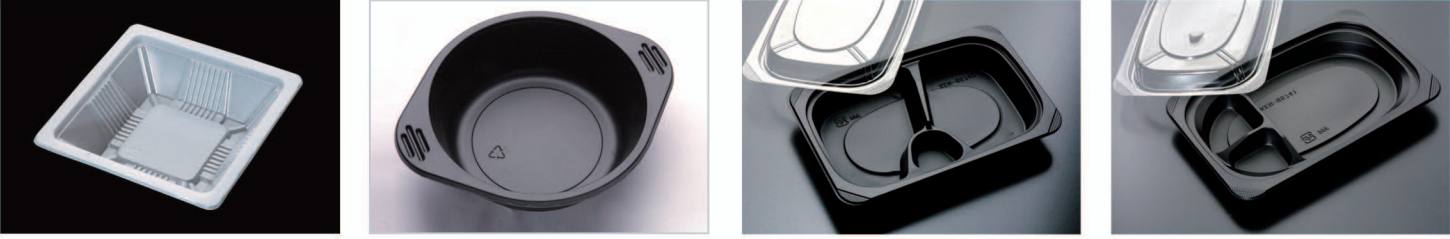
名 称:400G 模具编号: RZ-35 制品尺寸: 151×151×40 纸箱尺寸: 575×445×535 材质:PP 克重: 20g 入箱数: 900枚 名 称:PP洋葱球 模具编号: RZ-49 制品尺寸: 196×159×52 纸箱尺寸: 580×370×335 材质:PP 克重: 21g 每箱入数: 600枚 名 称:65740 模具编号: RZ-65S 制品尺寸: 226×150×37 纸箱尺寸: 1060×470×320 材质:盖OPS 身PP 克重: 17g 入箱数: 1000枚 名 称:65741 模具编号: RZ-65S 制品尺寸: 226×150×28. 5 纸箱尺寸: 980×470×320 材质:盖OPS 身PP 克重: 20g 入箱数: 1000枚
