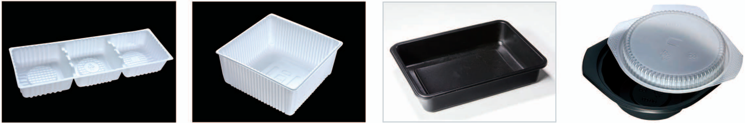
名称:趣多多80g 模具编号: RZ-116 制品尺寸: 191×65×26 纸箱尺寸: 600×570×410 材质:PP 克重: 3. 7g 入箱数: 4200枚 名称:太平苏打100g 模具编号: RZ-120 制品尺寸: 106×106×47 纸箱尺寸: 640×340×550 材质:PP 克重: 3g 入箱数: 3300枚 名称: PP黑色鱼块托盘 模具编号: RZ-129 制品尺寸: 179×129×35 纸箱尺寸: 575×445×534 材质:PP 克重: 18g 入箱数: 800枚 名称: RR-03面汤碗 模具编号: RZ-130 制品尺寸: 盖217×188×69 身215×186×24. 5 克重: 盖13g 身24g 材质:PP 克重: 盖1000枚 身1000枚
