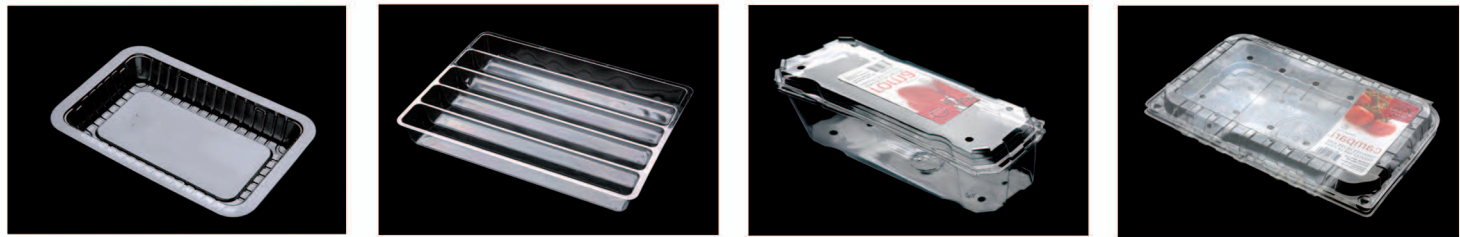
名称:2g海苔 模具编号:RZ-60 制品尺寸:110×71×15 纸箱尺寸:530×405×405 材质:PET 克重:1.5g 入箱数:7500枚 名称:五分格 模具编号:RZ-6 制品尺寸:201.5×147×28 纸箱尺寸:530×310×420 材质:PET 克重:14.5g 入箱数:1200枚 名称:ROMA盒 模具编号:RZ-55 制品尺寸:281×247×63 纸箱尺寸:545×515×590 材质:PET 克重:43g 入箱数:560枚 名称:2LB 模具编号:RZ-47 制品尺寸:380×285×41 纸箱尺寸:550×395×585 材质:PET 克重:45g 入箱数:330枚
