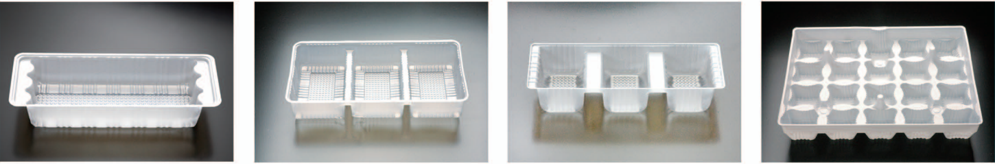
名 称:100g奶油饼干 材质:HIPS 模具编号: RZ-99 克重: 6.2g 制品尺寸: 200×76×40 入箱数: 1200枚 纸箱尺寸: 620×470×720 名 称:200g奶油饼干 材质:HIPS 模具编号: RZ-98 克重: 11.2g 制品尺寸: 221×118×40 入箱数: 800枚 纸箱尺寸: 690×470×630 名 称:120g奶油饼干 材质:HIPS 模具编号: RZ-100 克重: 5.8g 制品尺寸: 200×70×43 入箱数: 1650枚 纸箱尺寸: 620×470×730 名 称:20格冷冻混沌托盘 材质:HIPS 模具编号: RZ-71 克重: 32g 制品尺寸: 315.4×252.4×51.6 入箱数: 800枚 纸箱尺寸: 609×533×328
