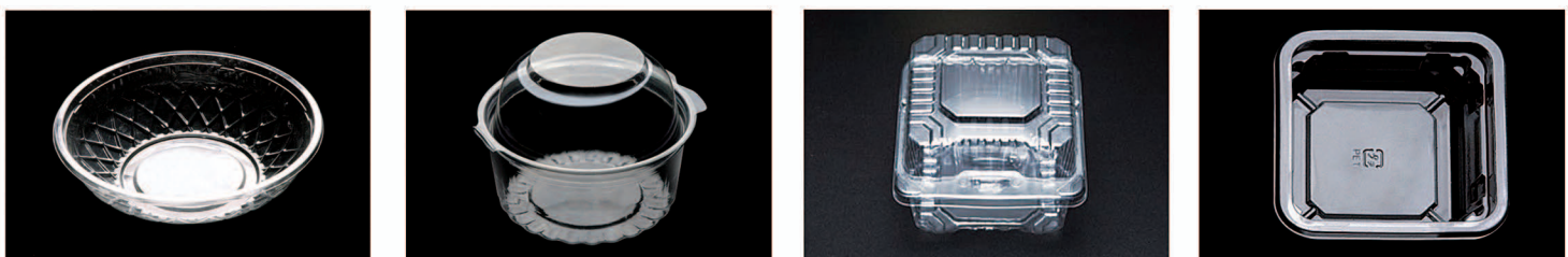
名称:FD-180碗 模具编号:RZ-78 制品尺寸:D180×51 纸箱尺寸:550×550×400 材质:PET 克重:15.4g 入箱数:400枚 名称:PET连体碗 模具编号:RZ-97 制品尺寸:245×118×(56+10) 纸箱尺寸:250×600×420 材质:PET 克重:15g 入箱数:250枚 名称:豆芽连体盒 模具编号:RZ-107 制品尺寸:229.3×112×61 纸箱尺寸:570×450×245 材质:PET 克重:13.8g 每箱入数:500枚 名称:海带丝盒 模具编号:RZ-34 制品尺寸:90×90×22 纸箱尺寸:720×555×470 材质:PET 克重:4.5g 每箱入数:3000枚
