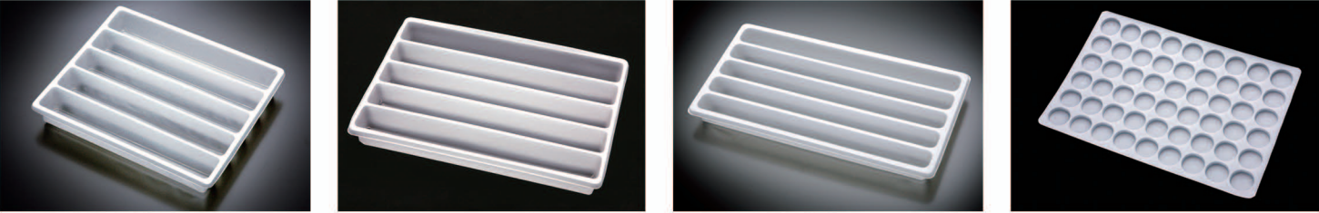
名 称:五分格25×25 模具编号: RZ-4 制品尺寸: 205×148×25 纸箱尺寸: 575×445×535 材质:PP 克重: 12. 5g 入箱数: 1250枚 名 称:五分格30×30 模具编号: RZ-56 制品尺寸: 206×174. 5×30 纸箱尺寸: 575×445×535 材质:PP 克重: 15g 入箱数: 1200枚 名 称:五分格17×20 模具编号: RZ-5 制品尺寸: 209×115×20 纸箱尺寸: 575×445×535 材质:PP 克重: 10. 9g 入箱数: 1440枚 名 称:菠菜容器 模具编号: RZ-17 制品尺寸: 379×270×10 纸箱尺寸: 530×405×405 材质:PP 克重: 58g 入箱数: 300枚
