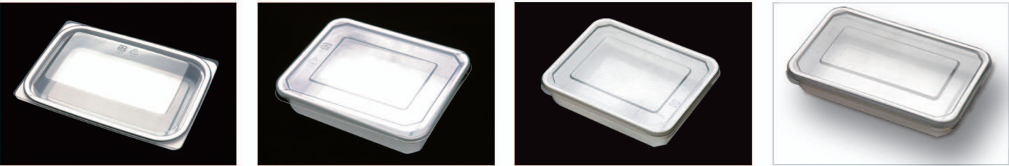
名 称:300G 材质:盖PET 身HIPS 模具编号: RZ-43 制品尺寸: 盖165×130×21 身185×130×25 纸箱尺寸: 盖520×340×370 身520×340×370 克重: 盖14.5g 身15.8g 入箱数: 盖400枚 身400枚 名 称:400g 材质:盖PET 身HIPS 模具编号: RZ-37 制品尺寸: 身155×155×32 盖161×161×10 纸箱尺寸: 盖640×420×490 身620×500×505 克重: 盖32g 身16g 入箱数: 盖600枚 身1350枚 名 称:160g 材质:盖PET 身HIPS 模具编号: RZ-36 制品尺寸: 盖135×108×10 身133×106×31 纸箱尺寸: 盖620×560×455 身550×455×555 克重: 盖10.3g 身14g 入箱数: 盖1000枚 身1600枚 名 称:200g地瓜盒 材质:盖PET 身HIPS 模具编号: RZ-75 制品尺寸: 盖156×116×9 身155×115×35 纸箱尺寸: 盖575×445×535 身575×445×535 克重: 盖12.7g 身18g 入箱数: 盖800枚 身1200枚
