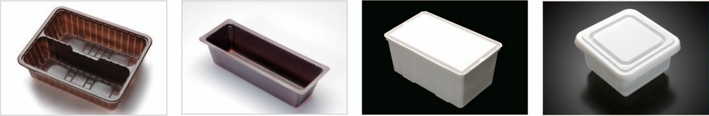
名 称:100g两联饼干 材质:HIPS 模具编号: RZ-15 克重: 10g 制品尺寸: 128×166 入箱数: 1200枚 纸箱尺寸: 550×530×510 名 称:90g饼干盒 材质:HIPS 模具编号: RZ-16 克重: 4.8g 制品尺寸: 177×64×31 入箱数: 3000枚 纸箱尺寸: 525×510×535 名 称:法国蛋糕 材质:HIPS 模具编号: RZ-51 制品尺寸: 盖208×120×10 身208×120×100 纸箱尺寸: 盖500×370×440 身580×455×350 克 重: 盖22.5g 身9.1g 入箱数: 盖400枚身800枚 名 称:冰激凌盒 材质:HIPS 模具编号: RZ-14 制品尺寸: 盖115×115×12 身110×110×85 纸箱尺寸: 盖580×350×464 身520×500×440 克 重: 盖12g 身15g 入箱数: 盖1000枚身600枚
