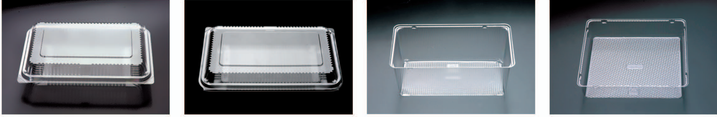
名 称:NO-3 材质:OPS 名 称:NO-4 材质:OPS 名 称:54#饼干 材质:OPS 名 称:35#饼干 材质:OPS 模具编号:RZ-82 模具编号:RZ-83 模具编号:RZ-112 模具编号:RZ-113 制品尺寸:260×190×35 克重:9.6g 制品尺寸:280×221×35 克重:13.5g 制品尺寸:137×78.5×51 克重:4.35g 制品尺寸:119.4×119.4×23.9 克重:2.8g 纸箱尺寸:560×395×600 入箱数:800枚 纸箱尺寸:800×570×450 入箱数:1000枚 纸箱尺寸:500×560×420 入箱数:1800枚 纸箱尺寸:500×550×390 入箱数:3600枚
