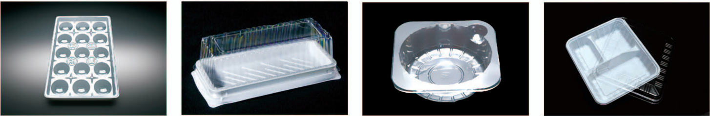
名 称:450g汤圆托盒 材质:OPS 名 称:三明治盒 材质:盖OPS 身HIPS 名 称:煎饼托盒 材质:OPS 名 称:餐盒盖 材质:OPS 模具编号:RZ-126 模具编号:RZ-124 模具编号:RZ-143 模具编号:RZR-05盖 制品尺寸:202×125×21 克重:4g 制品尺寸:盖163×74×43 身168×79×16 制品尺寸:85×85×24.6 克重:1g 制品尺寸:盖229×197×22 克重:7.1g 纸箱尺寸:575×445×535 入箱数:4500枚 克重:盖5g 身5.2g 身670×400×410 纸箱尺寸:盖660×470×390 入箱数:盖1000枚 身1000枚 纸箱尺寸:560×520×360 入箱数:12000枚 身尺寸:227×195×38 克重:28.7g
