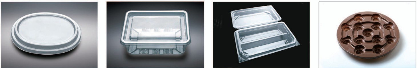
名称:PET盖子 模具编号:RZ-93 制品尺寸:125.5×100.5×13 纸箱尺寸:575×445×535 材质:PET 克重:5.5g 每箱入数:1500枚 名称:沙拉盒 模具编号:RZ-133 制品尺寸:身162×120.5×52 盖165×123.5×9 纸箱尺寸:身720×620×340 盖510×430×500 克重:身22g 盖14g 每箱入数:1000枚 材质:PET 克重:12g 每箱入数:900枚 名称:寿司卷连体盒 模具编号:RZ-139 制品尺寸:208×180×25 纸箱尺寸:635×470×550 材质:PET 克重:12g 每箱入数:900枚 名称:圆形巧克力 模具编号:RZ-170 制品尺寸:D173.5X20 纸箱尺寸:440X370X370 材质:PET 克重:12g 入箱数800枚
