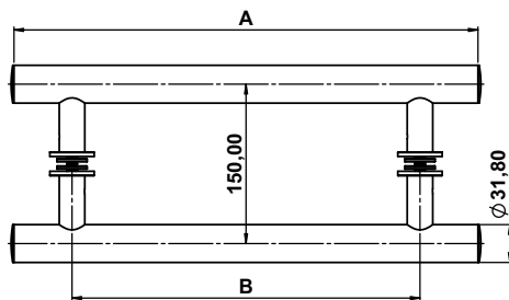
Par de Puxadores para Porta Redondo Preto Fosco Material: Alumínio
