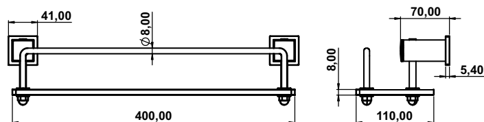
Porta Shampoo Square Semi-Luxo Preto Fosco COD.: 215315
