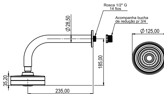
Ducha Autolimpante Q/F Preto Fosco - Abs C/Cano Inox Cód.: 216004
