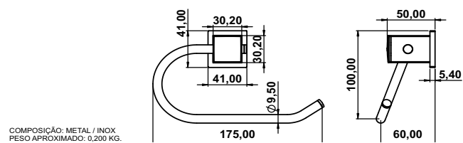
Papeleira Semi Luxo Square Inox Rose Fosco COD.: 214931
