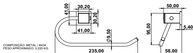
Porta Toalha Rosto Semi Luxo Square Rose Fosco COD.: 214933
