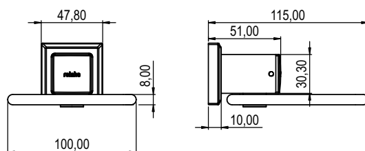
Porta Toalha Duplo Square em Aço Inox COD.: 212545
