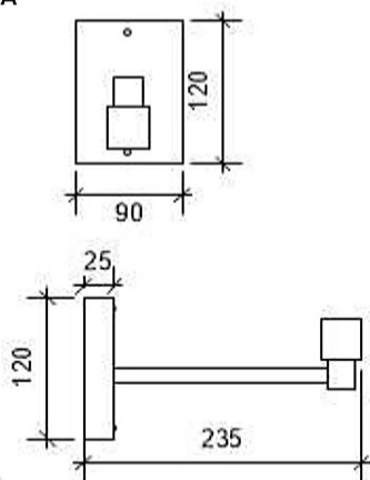
OPÇÃO CANOPLA NA VERTICAL
