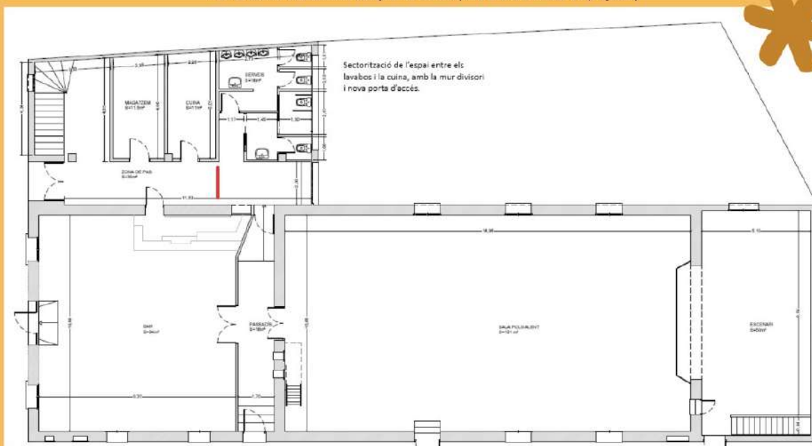
Planta Baixa: Actuacions complementàries (fora d'abast inicial de projecte)
