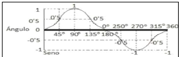
Figura 5. A cada ángulo (eje x) le corresponde un seno, un punto en la curva. Todos los puntos de la onda son senos de ángulos = \sin \alpha . (Imagen del autor).
