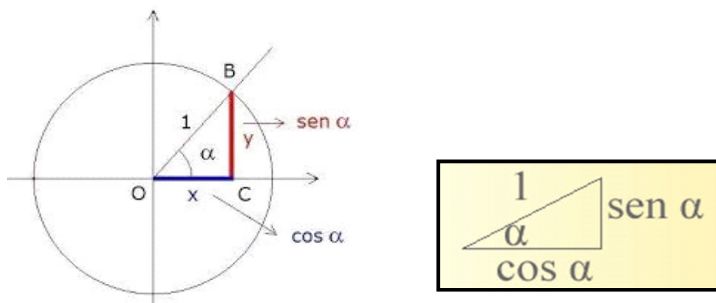
FIGURA 2. El seno de un ángulo por definición recordemos que es el cateto opuesto dividido por la hipotenusa. Hipotenusa que en la circunferencia unitaria vale 1. Por tanto, el seno es: y = \text{cateto opuesto dividido por hipotenusa } (1) = \text{seno} . Y es el sen de \alpha
