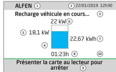
Figure 1 : Affichage de l'Eve Single Pro-line FR pendant la charge avec prise type 2
