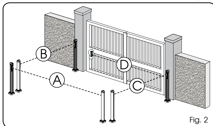
La fig. 2 illustre un automatisme pour portail battant à 2 vantaux avec les faisceaux de couverture des photocellules:
