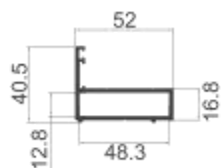
MQ-K01 开启框 壁厚: 2.0 mm 米重: 0.88 kg/m
