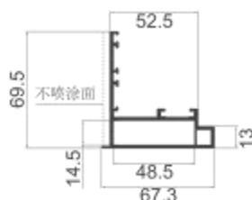
MQ-K02 隐框开启扇 壁厚: 2.0 mm 米重: 1.34 kg/m
