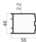
DTM01 光企 壁厚: 2.2 mm 米重: 1.21 kg/m
