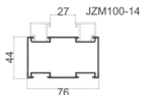
JH-GD01 隔断中柱 壁厚: 1.4 mm 米重: 1.087 kg/m
