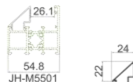
JH-M5504 压线 壁厚: 1.0 mm 米重: 0.192 kg/m
