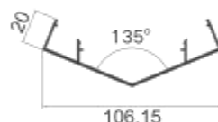
MQ-M13 明135度阳转角压板 壁厚: 1.6 mm 米重: 0.73 kg/m
