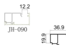
JH-068 框压线 壁厚: 1.0 mm 米重: 0.311 kg/m
