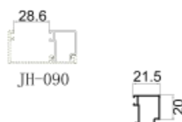
JH-6805 方压线 壁厚: 1.0 mm 米重: 0.222 kg/m
