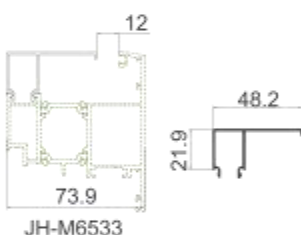
JH-M6515A 外开扇压线 壁厚: 1.1 mm 米重: 0.336 kg/m
