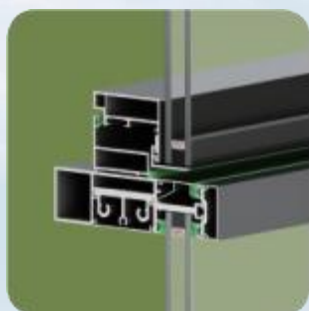
橫面型材
