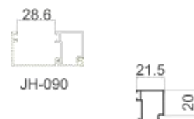
JH-6805 方压线 壁厚: 1.0 mm 米重: 0.222 kg/m
