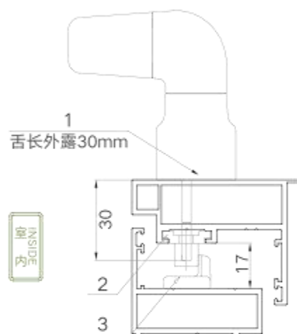
执手, 传动杆, 中间锁块节点图
