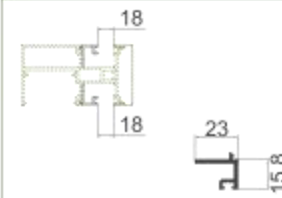
MQ-M20 明框单玻转换料 壁厚: 2.0 mm 米重: 0.27 kg/m
