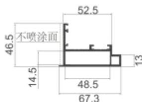
MQ-K04 明框开启扇 壁厚: 2.0 mm 米重: 1.17 kg/m
