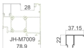
JH-M6511 压线 壁厚: 1.1 mm 米重: 0.303 kg/m
