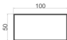
100x50 方管 壁厚: 2.0 mm 米重: 1.59 kg/m
