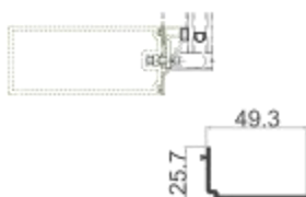
MQ-K03 隐框开启收边 壁厚: 2.0 mm 米重: 0.41 kg/m
