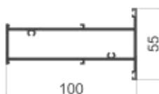
MQ-M33 100中柱 壁厚: 2.0 mm 米重: 1.637 kg/m
