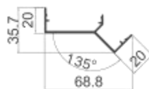
MQ-M17 明135度阴转角压盖 壁厚: 1.6 mm 米重: 0.45 kg/m
