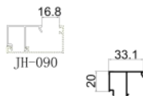
JH-M12027 框压线 壁厚: 1.2 mm 米重: 0.301 kg/m
