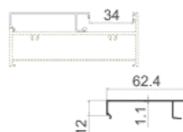
MQ-M34 压线 壁厚: 1.1 mm 米重: 0.299 kg/m
