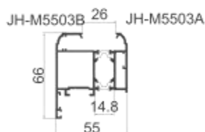
JH-M5503 玻扇 壁厚: 1.1 mm 米重: 1.365 kg/m
