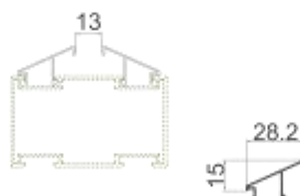
JH-GD03 斜压线 壁厚: 0.8 mm 米重: 0.14 kg/m
