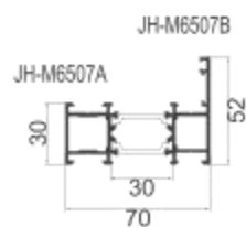
JH-M7007 外框 壁厚: 1.35 mm 米重: 1.277 kg/m
