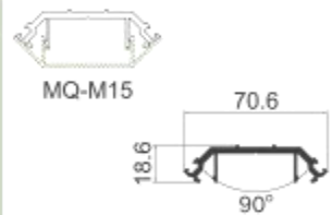
MQ-M14 明90度阴转角压板 壁厚: 3.0 mm 米重: 0.81 kg/m
