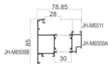
JH-M7009 窗扇 壁厚: 1.35 mm 米重: 1.632 kg/m
