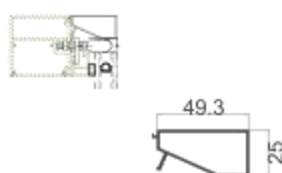
MQ-Y09 隐框收边 壁厚: 1.4 mm 米重: 0.53 kg/m
