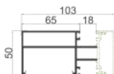
MQ-M28 明框横梁 壁厚: 1.9 mm 米重: 1.366 kg/m
