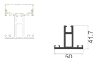
MQ-M31 50底座 壁厚: 3.0 mm 米重: 1.188 kg/m
