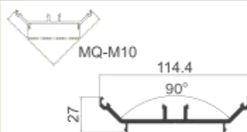
MQ-M09 明90度阳转角压板 壁厚: 3.0 mm 米重: 1.27 kg/m
