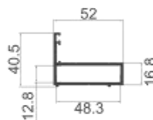
MQ-K01 开启框 壁厚: 2.0 mm 米重: 0.88 kg/m
