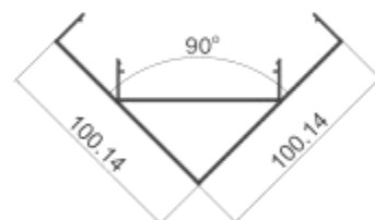
MQ-M10 明90度阳转角压盖 壁厚: 1.6 mm 米重: 1.48 kg/m
