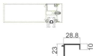
MQ-M07 明框开启收边 壁厚: 2.0 mm 米重: 0.32 kg/m
