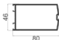
DTM04 光企 壁厚: 2.2 mm 米重: 1.505 kg/m
