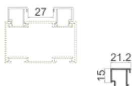
JZM100-14 方压线 壁厚: 1.2 mm 米重: 0.22 kg/m
