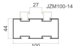
JH-GD02 隔断中柱 壁厚: 1.4 mm 米重: 1.264 kg/m
