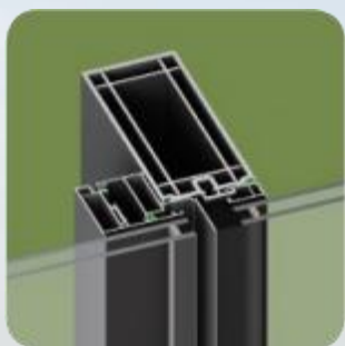
豎面型材
