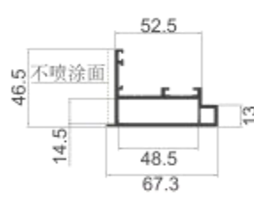
MQ-K04 明框开启扇 壁厚: 2.0 mm 米重: 1.17 kg/m
