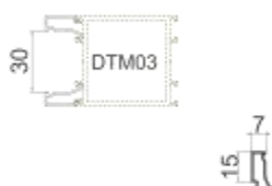
DTM05 双玻压线 壁厚: 1.0 mm 米重: 0.13 kg/m
