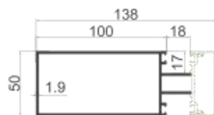
MQ-M27 100立柱 壁厚: 1.9 mm 米重: 1.803 kg/m
