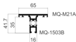
MQ-M21 65断桥底座 壁厚: 3.0 mm 米重: 0.92 kg/m
