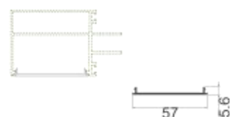
MQ-M6501 横梁盖板 壁厚: 1.2 mm 米重: 0.22 kg/m
