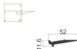
MQ-Y15 隐框玻璃托 壁厚: 3.5 mm 米重: 0.69 kg/m
