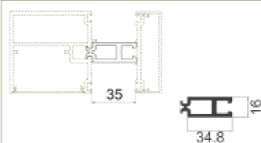
MQ-M19 隐转明辅料 壁厚: 2.5 mm 米重: 0.78 kg/m
