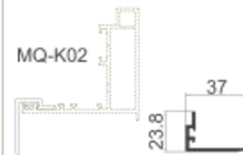
MQ-K06 开扇玻璃托 壁厚: 2.0 mm 米重: 0.36 kg/m
