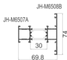
JH-M7008 中框 壁厚: 1.35 mm 米重: 1.375 kg/m
