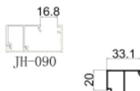
JH-M12027 框压线 壁厚: 1.2 mm 米重: 0.301 kg/m
