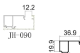
JH-068 框压线 壁厚: 1.0 mm 米重: 0.311 kg/m
