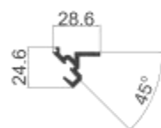
MQ-Y12 90度阳转角辅料 壁厚: 2.5 mm 米重: 0.42 kg/m
