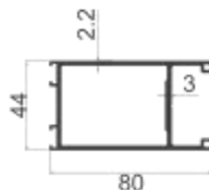
DTM02 上下方 壁厚: 2.2 mm 米重: 1.54 kg/m
