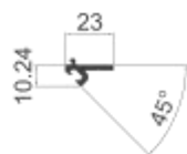
MQ-M08 明90度阳转角辅料 壁厚: 2.5 mm 米重: 0.25 kg/m
