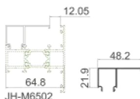
JH-M6505A 外开扇压线 壁厚: 1.1 mm 米重: 0.339kg/m
