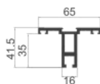
MQ-M01 65底座 壁厚: 3.0 mm 米重: 1.34 kg/m
