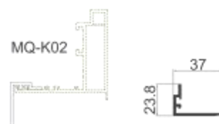
MQ-K06 开扇玻璃托 壁厚: 2.0 mm 米重: 0.36 kg/m
