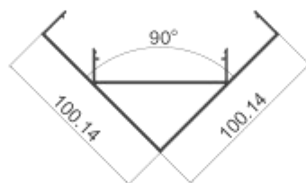
MQ-M10 明90度阳转角压盖 壁厚: 1.6 mm 米重: 1.48 kg/m
