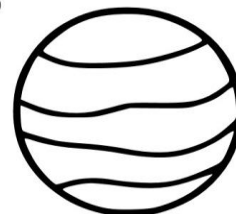
URANUS
