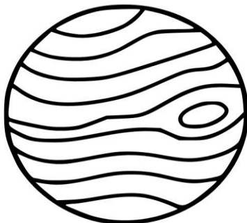
JUPITER
