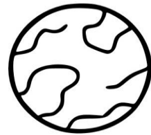
VENUS
