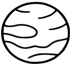
MARS
