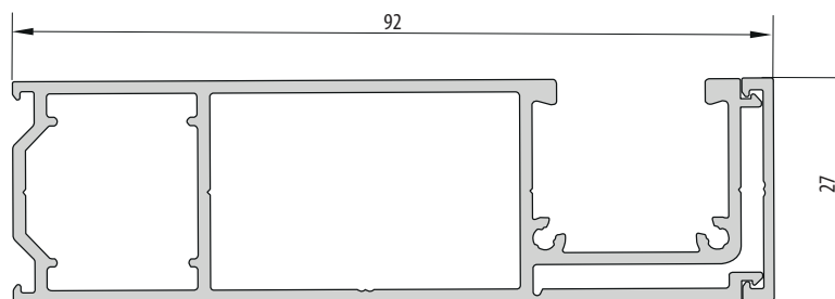
Coulisse monobloc Eko-Okna
