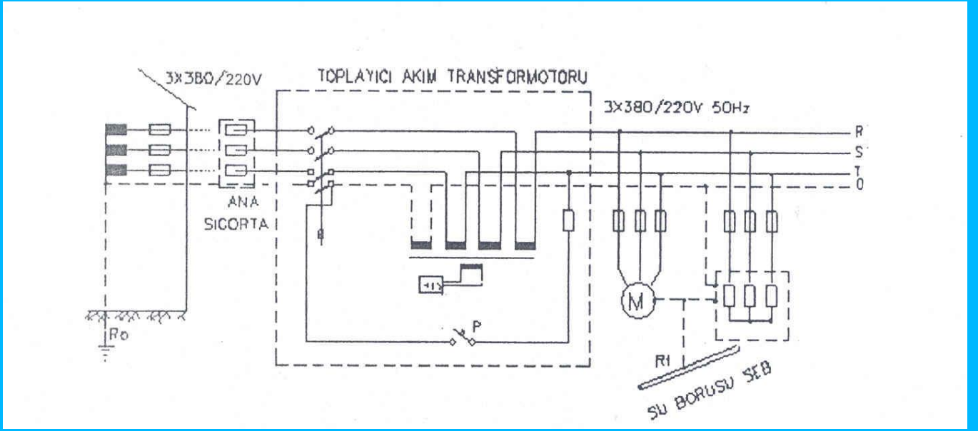
Şekil - 17 Hata akımı koruma bağlaması
