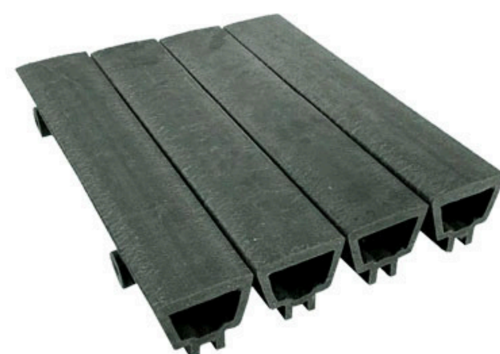
PÍER MARÍTIMO 400x90mm PESO: 47 Kg/m
