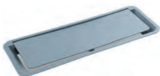
Trappes ABS sans nourrice Pour plateaux ép. 19 mm ABS injecté blanc OG, gris aluminium OI ou noir OF (+ fin.)
