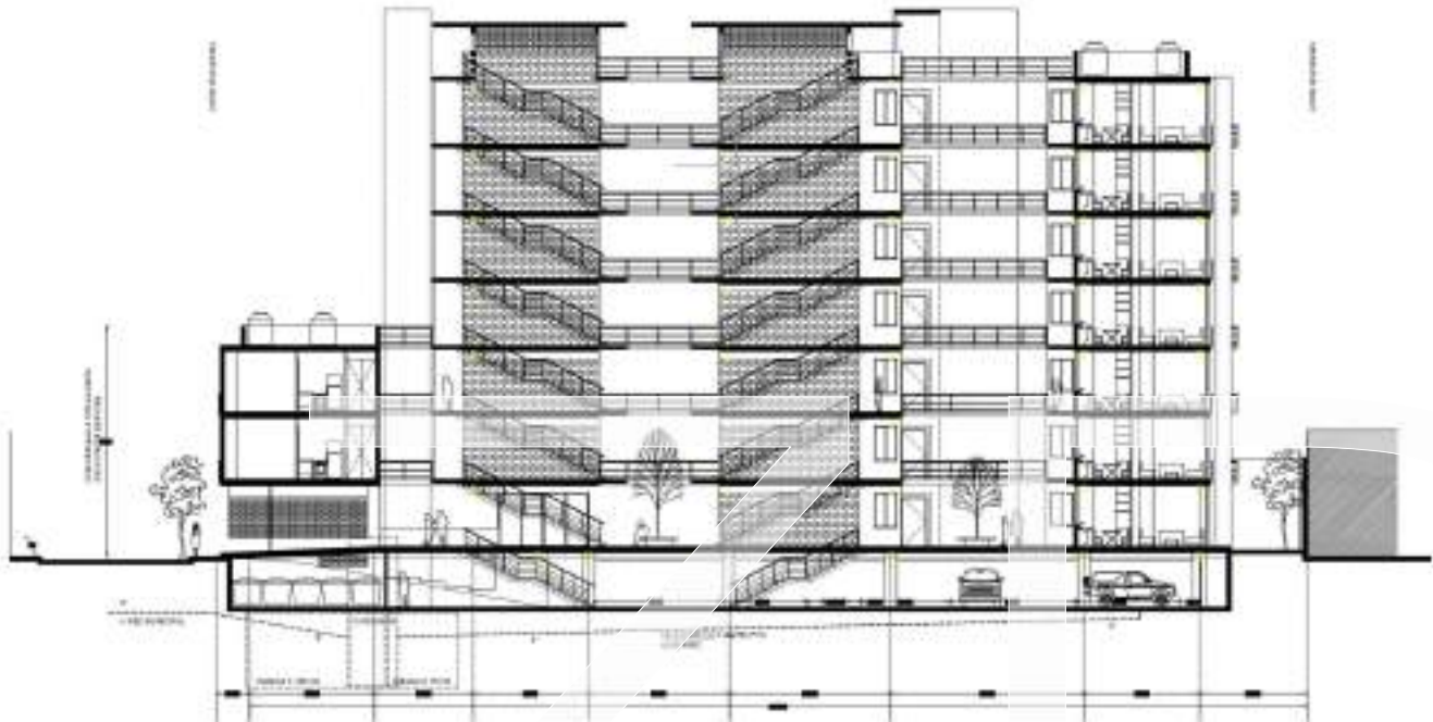
Secciones.
