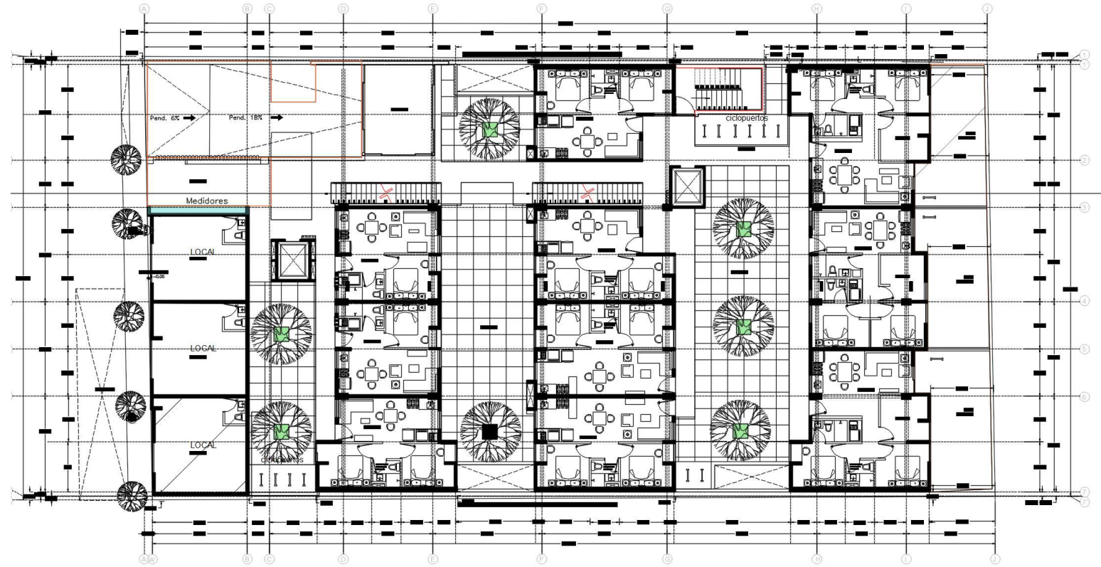
NIVEL PLANTA BAJA | NIVEL ± 0.48
