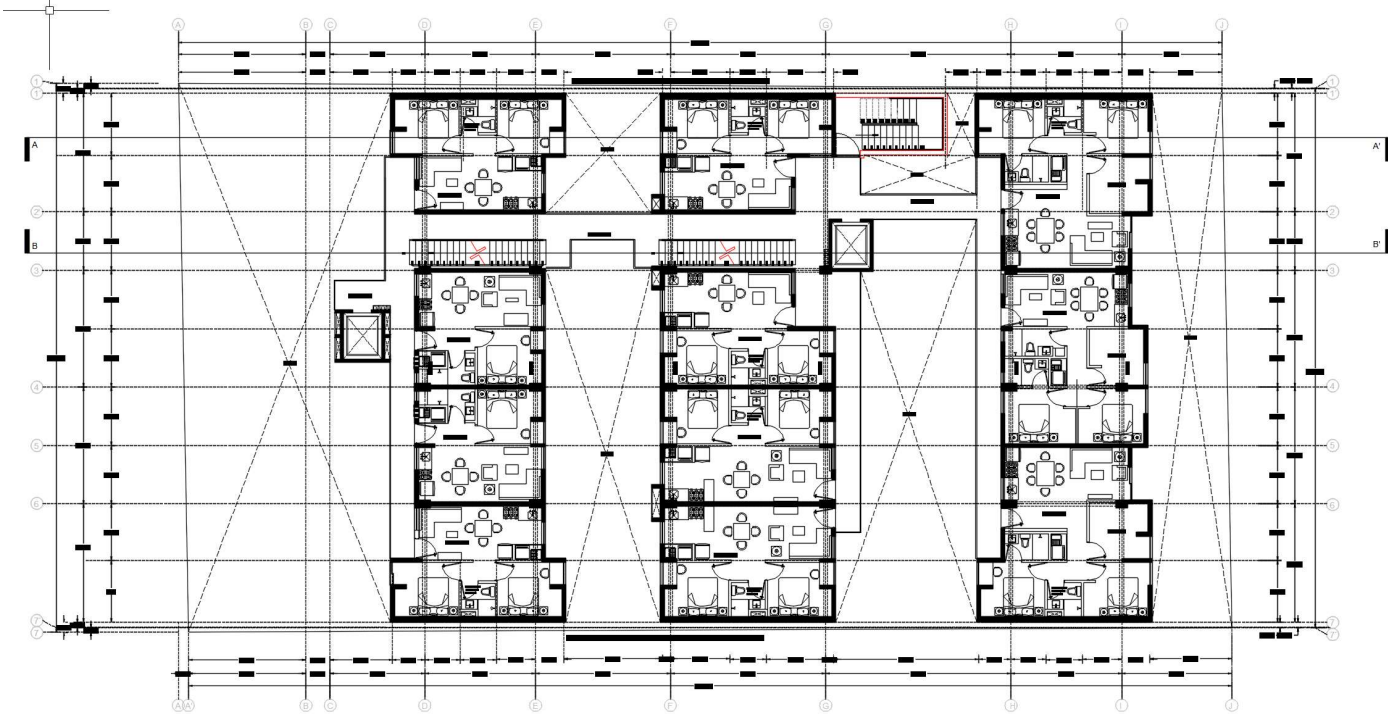
PLANTA NIVEL 6 | NIVEL +19.68
