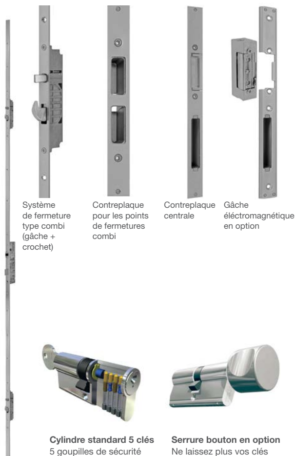
Verrou à bascule (crochet) et verrou automatique qui se ferment en tandem
