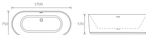
SAYA FLOORSTANDING BATH
