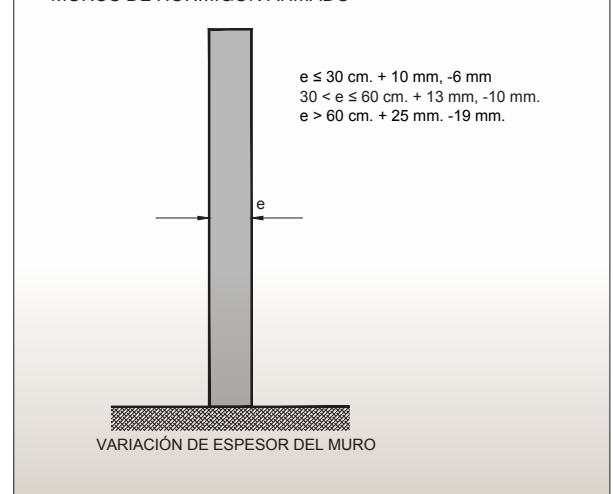
FIGURA 1. MUROS DE HORMIGÓN ARMADO
