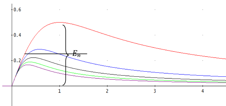
Gráficos de algunas f_n
