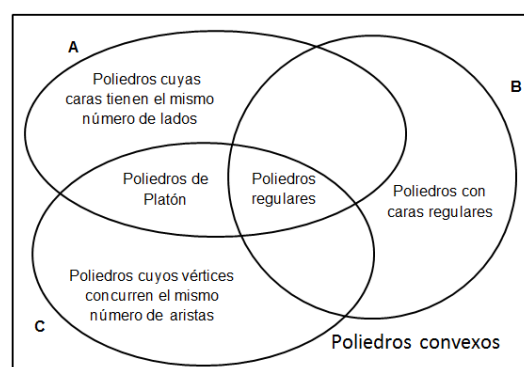
Figura 1 Poliedros convexos, de Platón y regulares.
