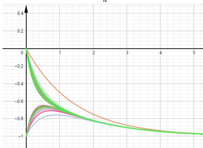
Gráficos de algunas sumas parciales de la serie.
