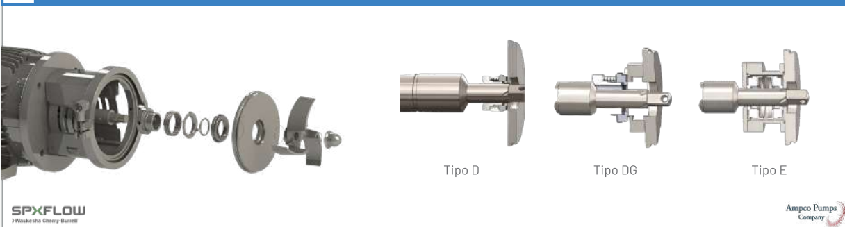
2. Opciones de sellado
