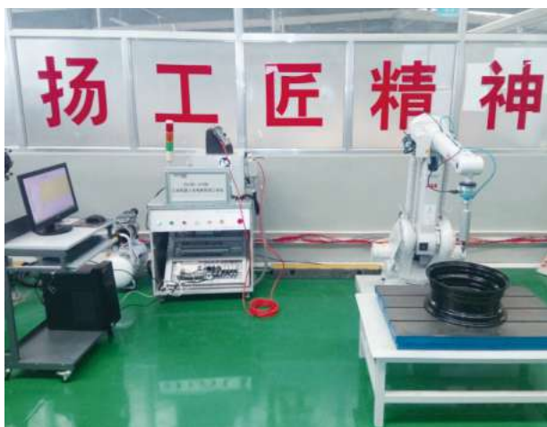
DLRB-1410B 工业机器人去毛刺实训工作站 Industrial Robot Deburring Training Workstation
