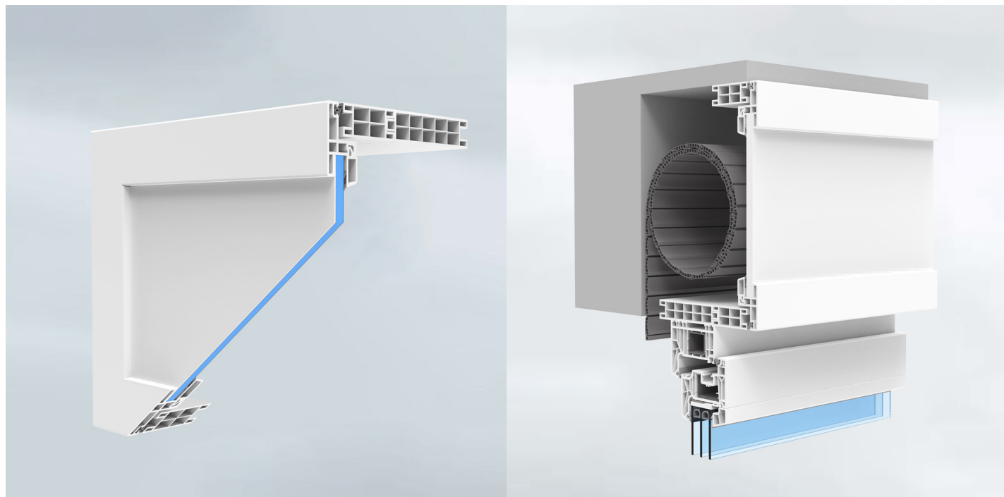
Sistema Schüco Cassonetto Easy Box
