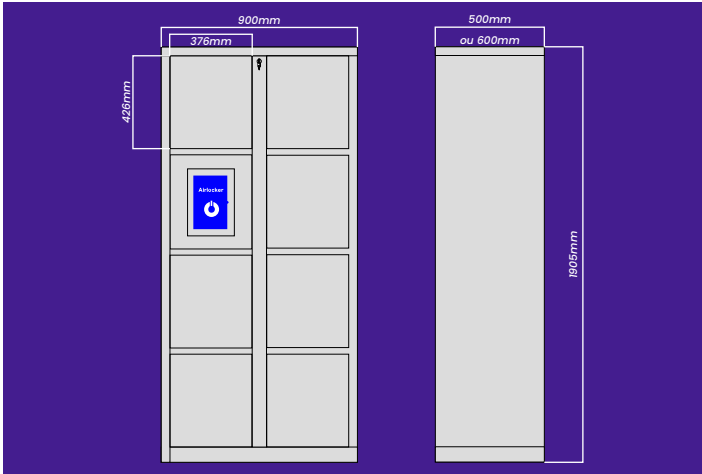
2 Armário Principal de 7 Portas 7 Portas médias
