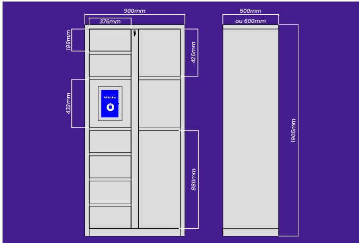
3 Armário Principal de 9 Portas 6 Portas pequenas 2 Portas médias 1 Porta grande
