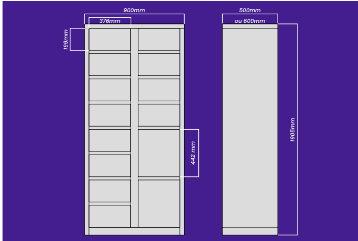
7 Armário Auxiliar de 14 Portas 12 Portas pequenas 2 Portas médias
