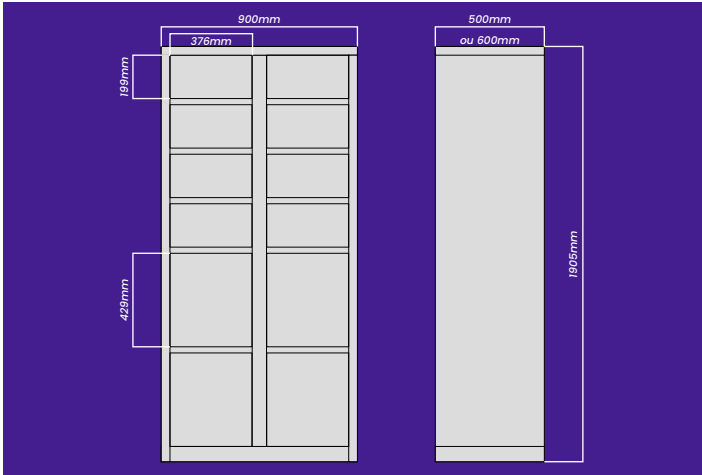
6 Armário Auxiliar de 12 Portas 8 Portas pequenas 4 Portas médias
