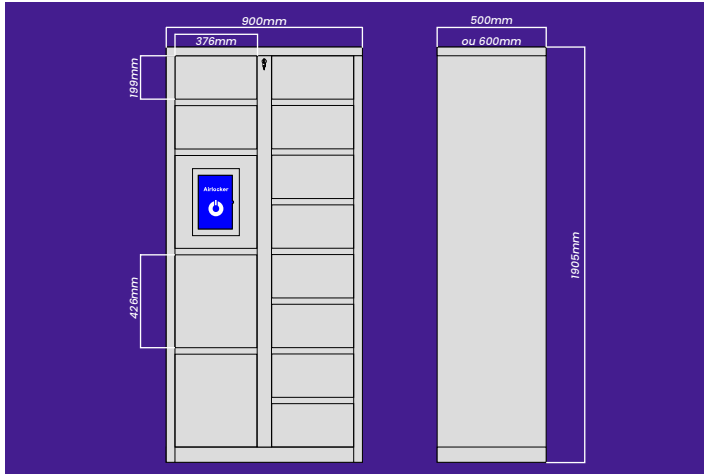
7 Armário Principal de 12 Portas Modelo 2 10 Portas pequenas 2 Portas médias
