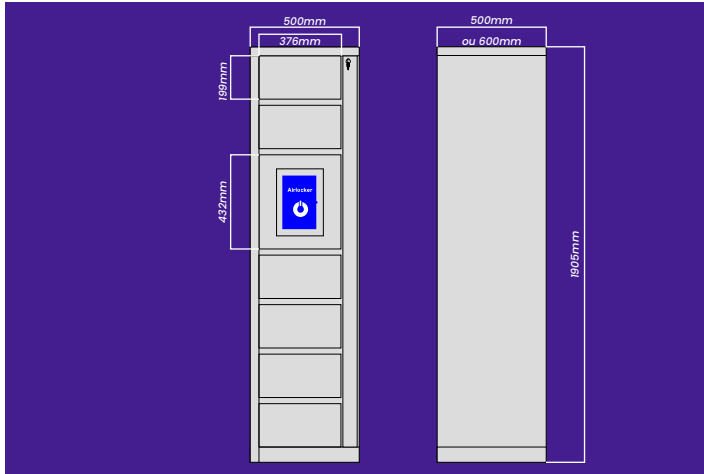
1 Armário Principal de 6 Portas 6 Portas pequenas
