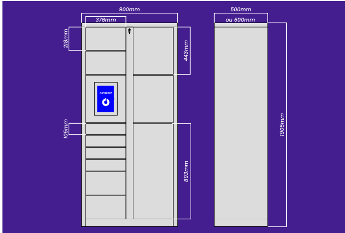
5 Armário Principal de 11 Portas 4 Portas PP 4 Portas pequenas 2 Portas médias 1 Porta grande
