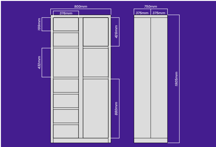
10 Armário Auxiliar Duplo de 10 Portas 6 Portas pequenas 3 Portas médias 1 Porta grande
