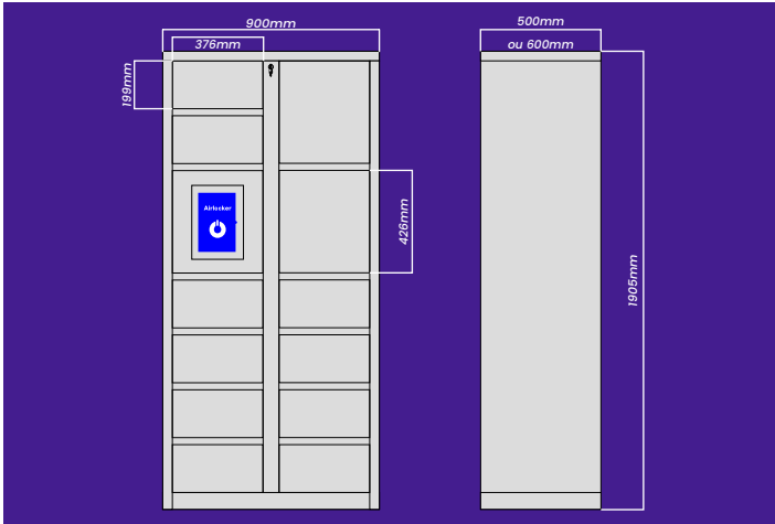
6 Armário Principal de 12 Portas Modelo 1 10 Portas pequenas 2 Portas médias
