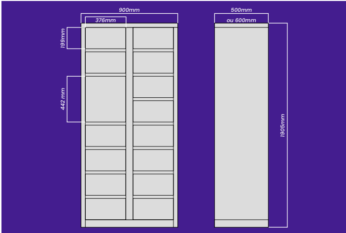
8 Armário Auxiliar de 15 Portas 13 Portas pequenas 1 Porta média
