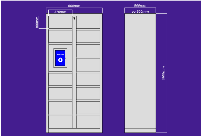
8 Armário Principal de 14 Portas 14 Portas pequenas
