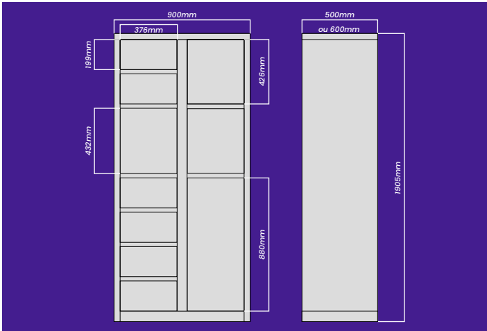
4 Armário Auxiliar de 10 Portas 6 Portas pequenas 3 Portas médias 1 Porta grande
