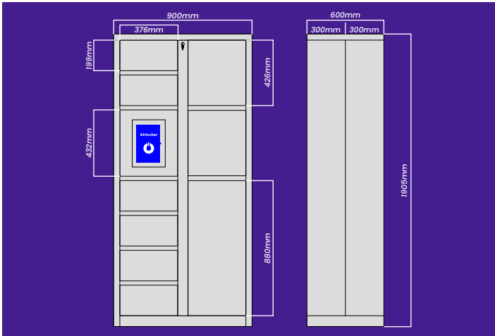
4 Armário Principal Duplo de 9 Portas 6 Portas pequenas 2 Portas médias 1 Porta grande
