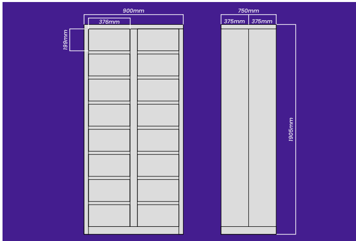
11 Armário Auxiliar Duplo de 16 Portas 16 Portas pequenas
