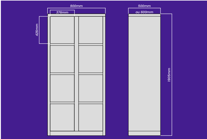
2 Armário Auxiliar de 8 Portas 8 Portas médias
