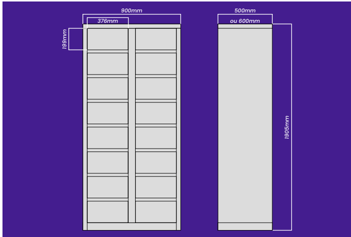
9 Armário Auxiliar de 16 Portas 16 Portas pequenas
