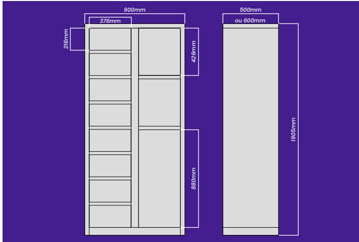
5 Armário Auxiliar de 11 Portas 8 Portas pequenas 2 Portas médias 1 Porta grande
