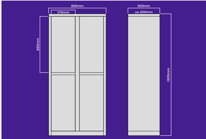
1 Armário Auxiliar de 4 Portas 4 Portas grandes
