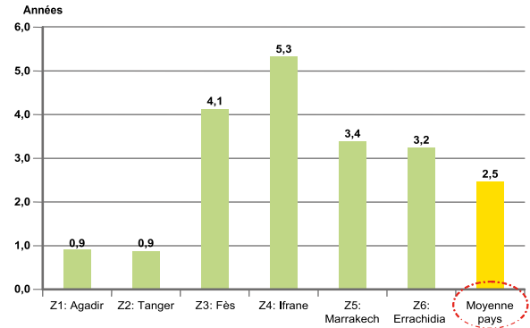
Figure 18 Temps de retour pour le consommateur final selon la zone climatique : bâtiments administratifs.
