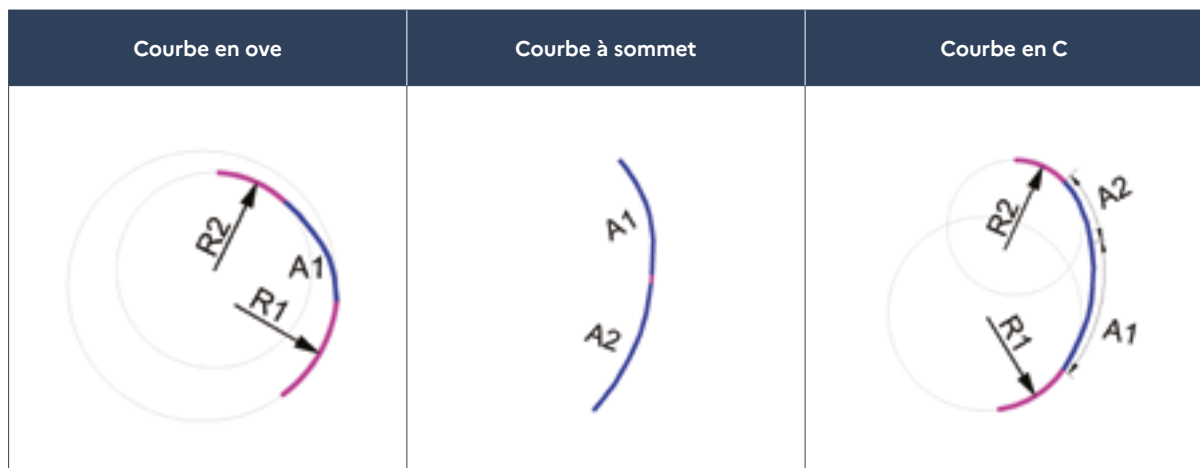
Figure 52 : Configurations de courbes à proscrire
