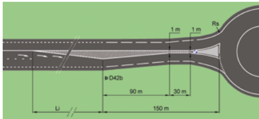
Figure 47 : Approche d'un giratoire depuis une artère interurbaine, avec entrée à 2 voies 169
