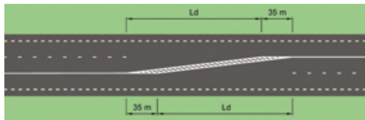
Figure 18 : Transition de créneaux divergents
