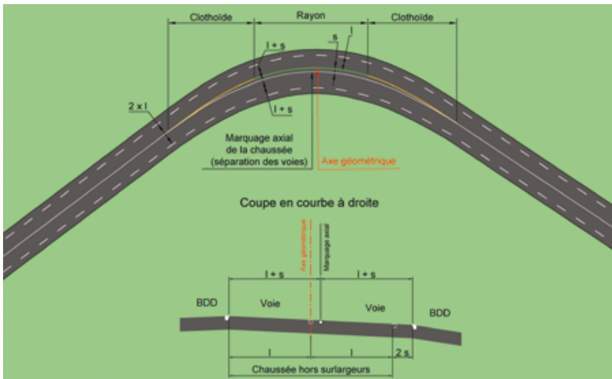
Figure 51 : Application des surlargeurs sur chaque bord de voie intérieur à la courbe
