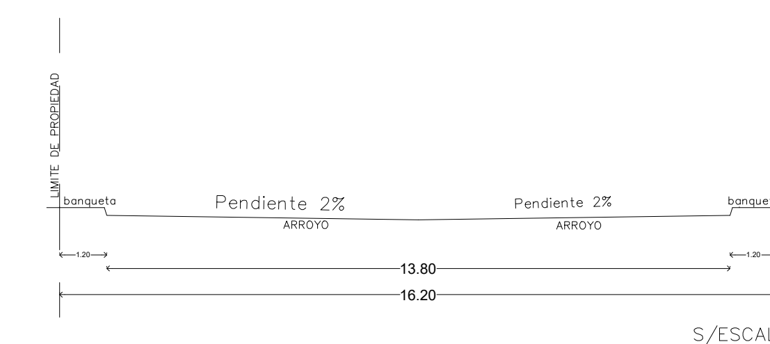
SECCION A-A'
