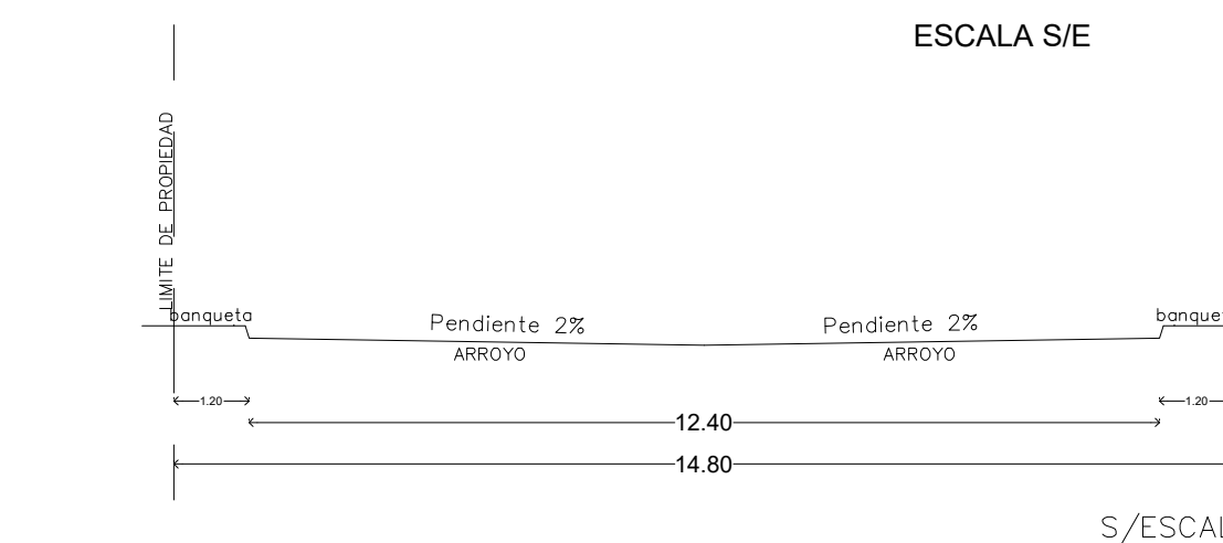
SECCION B-B'
