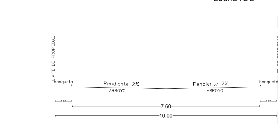
SECCION C-C'
