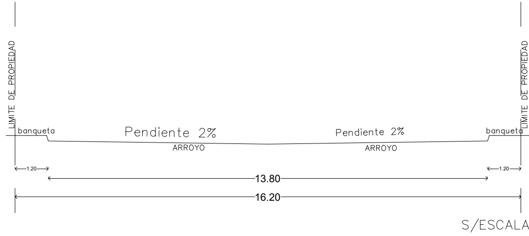
SECCION A-A'
