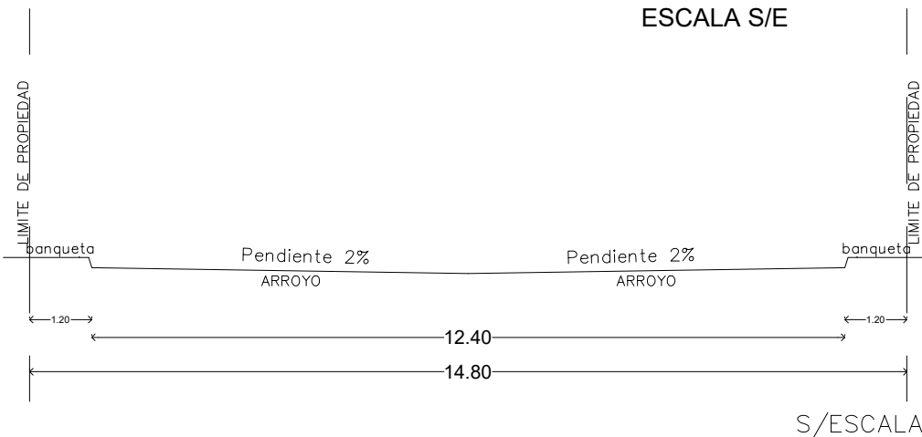
SECCION B-B'
