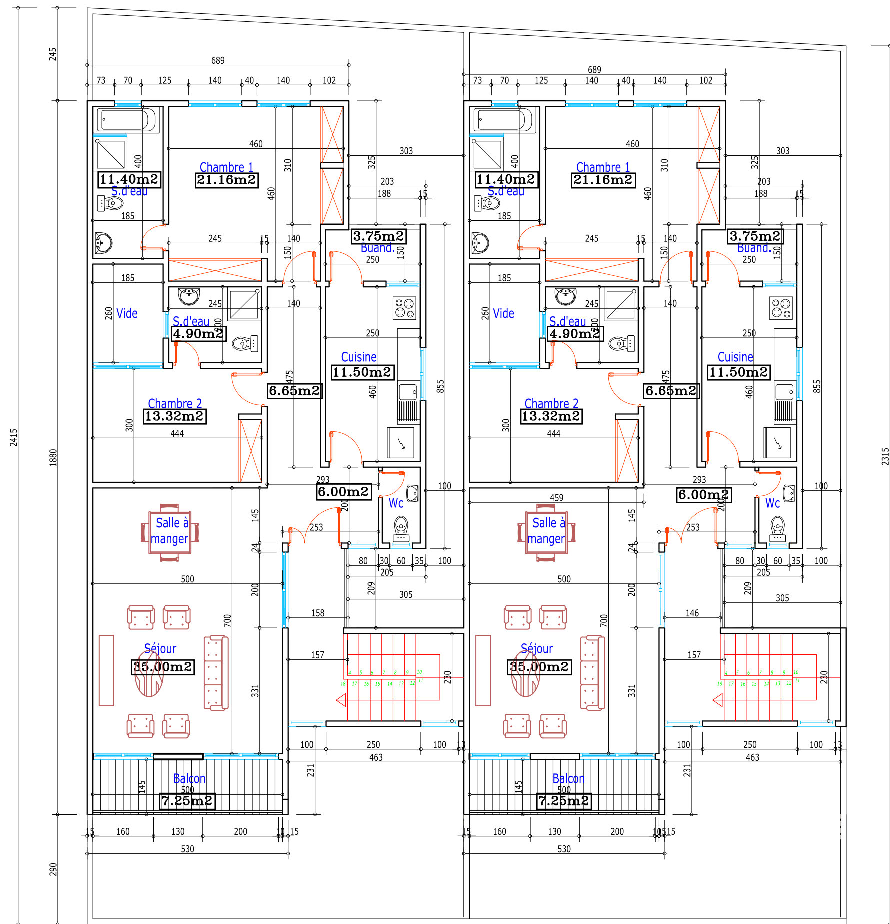
R+1 2 APPARTEMENTS DE 3PIECES (X 2) ETAGE
