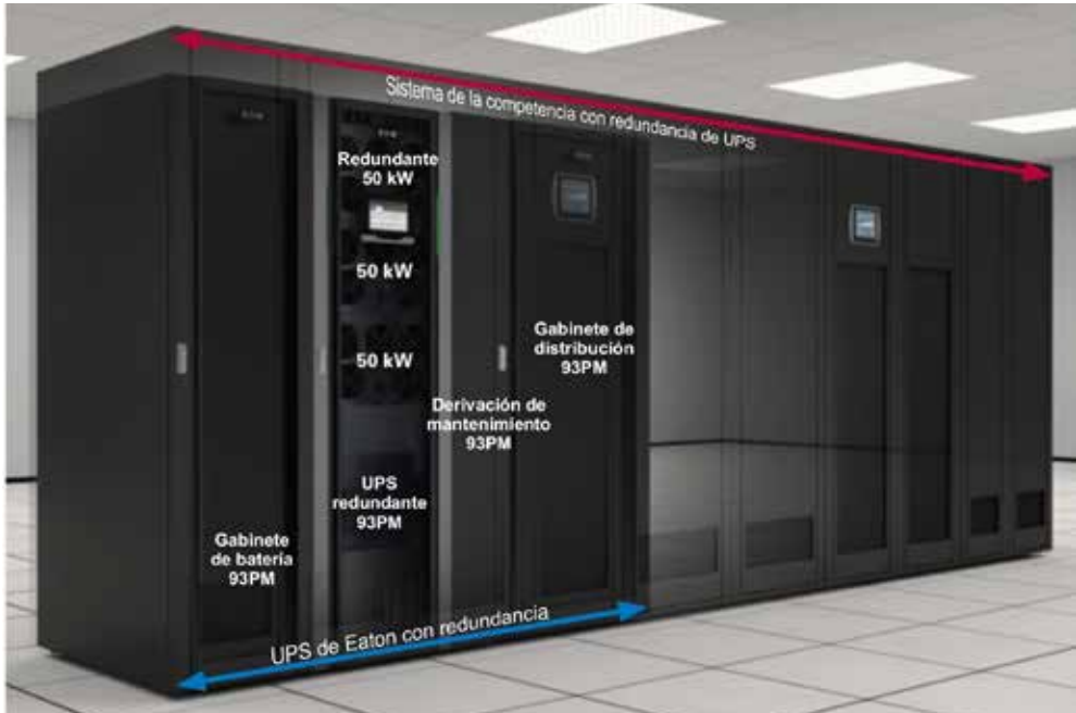
Diseño de espacio ocupado pequeño, redundancia interna y escalabilidad vertical del 93PM
